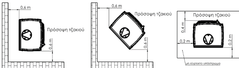
Σχ.3. Ασφαλείς αποστάσεις από το τζάκι
