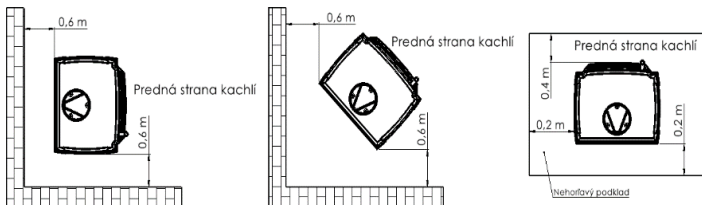
Obr.3. Bezpečné vzdialenosti od kachlí
