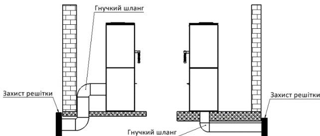
Рис. 2. Схема підключення подачі повітря
