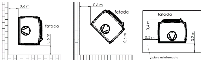
Fig.3. Distanța minimă de siguranță
