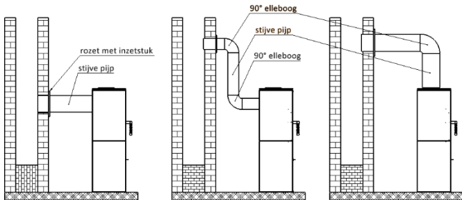
Afb. 4. Aansluitschema van de haard
