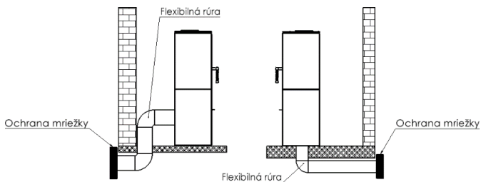
Obr. 2. Schéma pripojenia prívodu vzduchu
