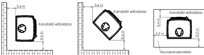
3 sz. Rajz. Biztonsági távolságok a kandallótól
