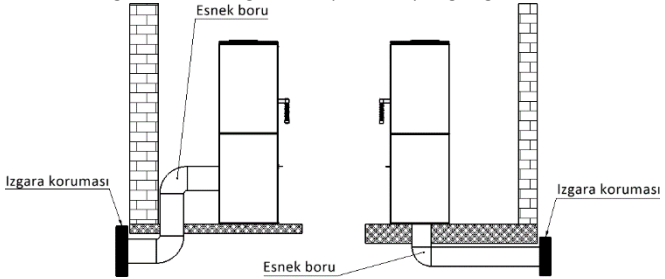
Şek. 2. Hava besleme bağlantısının şeması
