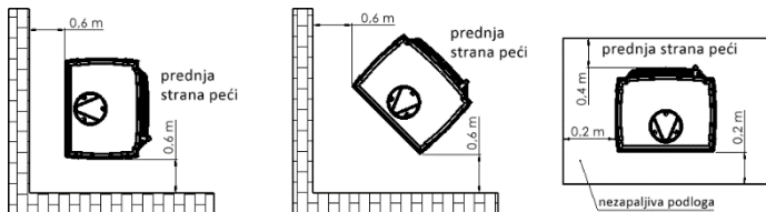
Crtež 3. Sigurna udaljenost od peći
