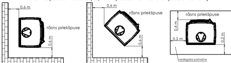
Att. 3 Droši attālumumi no krāsns
