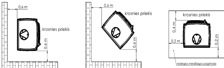
3 pav. Saugus atstumas nuo krosnies
