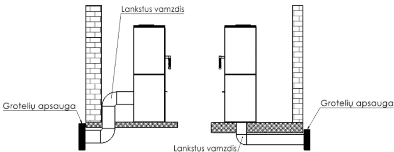
2 pav. Oro tiekimo jungties schema
