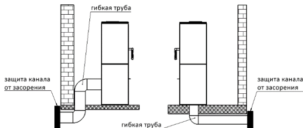
Рис. 2. Схема подключения подачи воздуха
