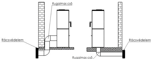
2 sz. Rajz. A levegőellátás csatlakozásának rajza
