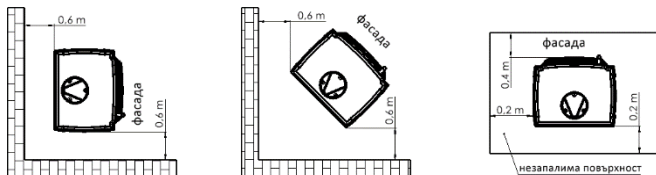
Фиг. 3. Безопасно разстояние от печката
