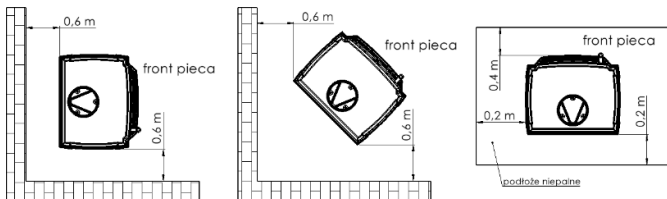
Rys.3. Bezpieczne odległości do pieca
