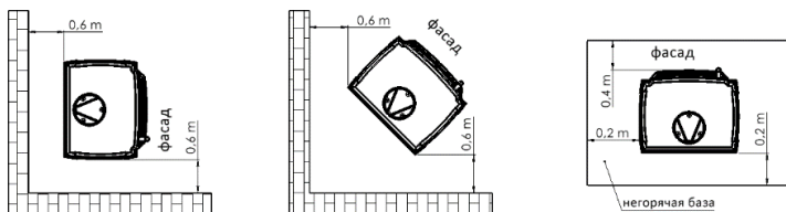
Рис. 3. Безопасное расстояние от печи
