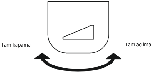
Şek. 4. Havanın hazneye erişiminin ayar örneği (küllük cephesinin görünümü).
