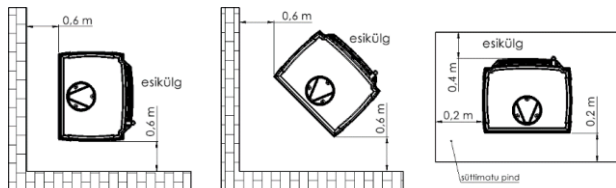
Joonis 3. Ohutu kaugus kaminast
