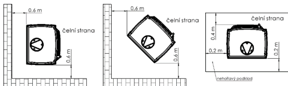
Obr. 3. Bezpečná vzdálenost od kamen
