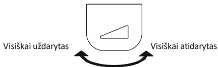
5 pav. Pavyzdinis oro padavimo į krosnį reguliavimas (peleninės fasado vaizdas).
