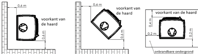
Afb. 3. Veilige afstand tot de haard
