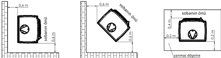
Şek. 3. Sobadan güvenli mesafeler
