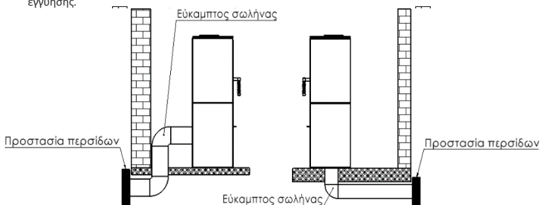
Σχ. 2. Διάγραμμα σύνδεσης παροχής αέρα
