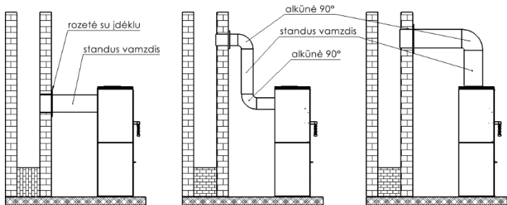
4 pav. Židininės krosnelės prijungimo schema
